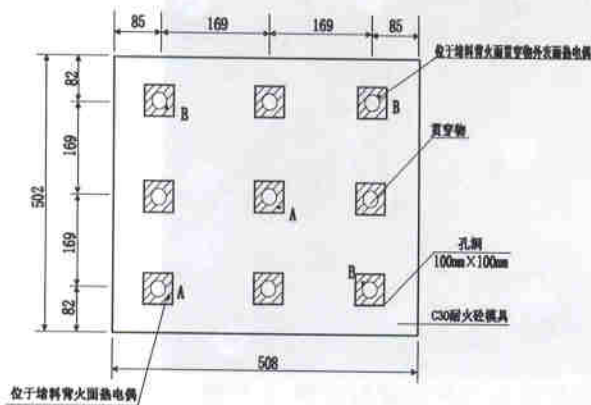
有机防火堵料耐火试验安装图
