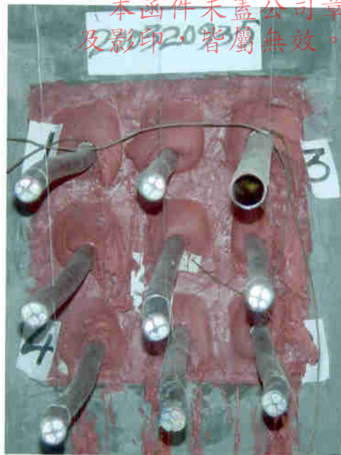
照片2 耐火试验结束时试件情况
